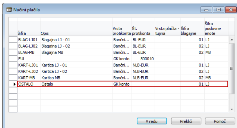
Slika 3: Načini plačila
