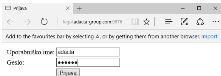
Slika 6: Prijava
